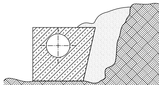
Figura 10-7 Punto de interferencia entre el macizo de anclaje y el suelo sólido
