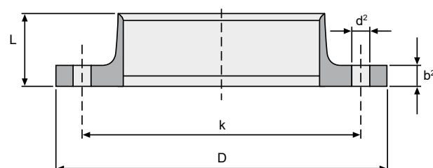
Figura 8-5 Brida fija
