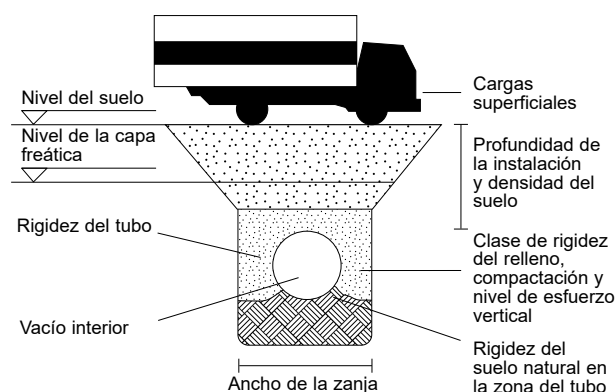
Figura 10-1 Parámetros aplicables al diseño de la instalación
