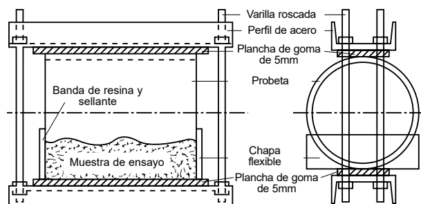
Figura 5-1 Equipo para medir el alargamiento unitario
