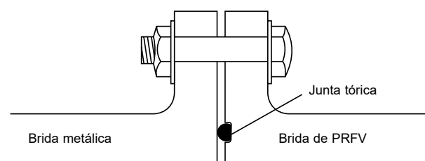
Figura 8-4 Unión por bridas
