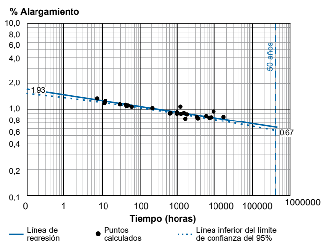
Figura 5-2 Línea Flowtite de alargamiento unitario
