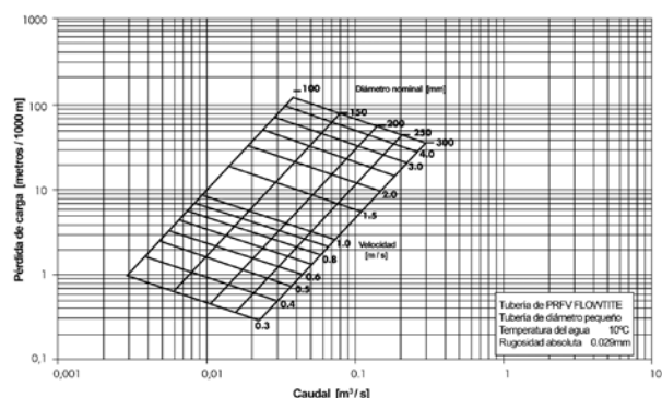
Figura 6-2 Pérdida de carga – diámetros pequeños
