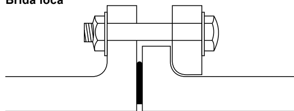
Figura 8-6 Brida loca con junta de goma con inserto de acero
