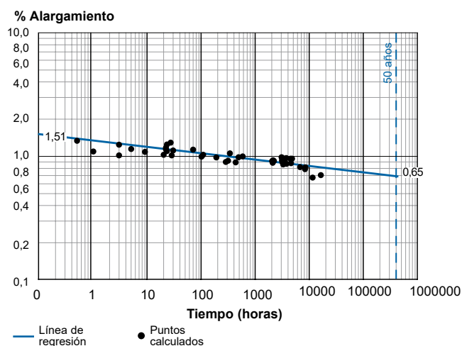
Figura 5-4 Línea Flowtite de alargamiento por presión a largo plazo
