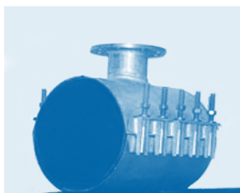
Figura 10-11 Mangas de toma recomendadas para uso con tubos de PRFV
