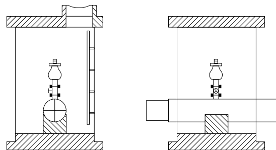
Figura 10-2 Cámaras de válvulas
