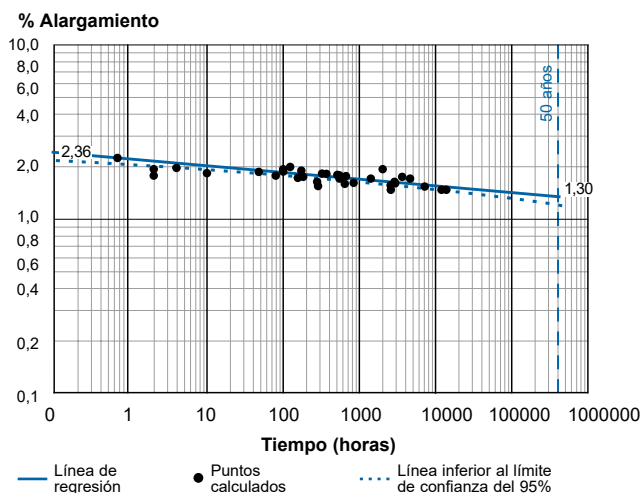
Figura 5-6 Línea Flowtite de deflexión a largo plazo
