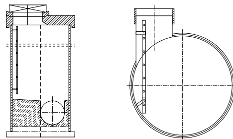
Figura 10-3 Pozo estándar y tangencial
