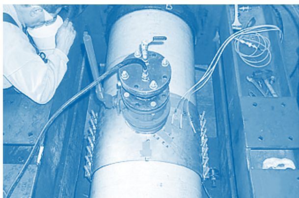
Figura 10-12 Ensayo de presión de la unidad manga-válvula
