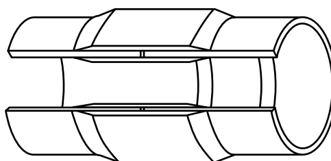
Figura 8-9 Unión por laminación química
