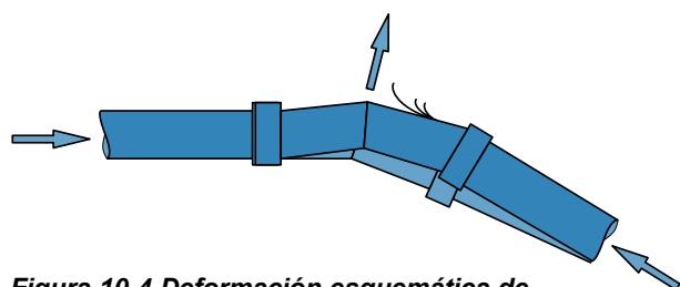
Figura 10-4 Deformación esquemática de accesorios inducida por fuerzas de empuje
