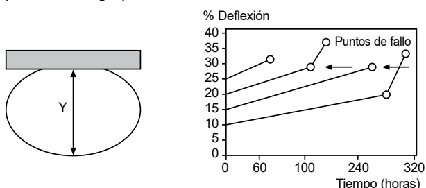
Figura 5-5 Efecto de la deflexión a largo plazo en una solución acuosa sobre la vida del tubo
