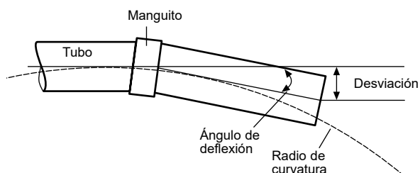
Figura 8-3 Desviación angular y radio de curvatura de la junta
