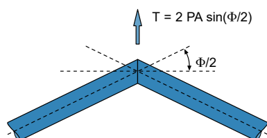
Figura 10-9 Fuerza de empuje
