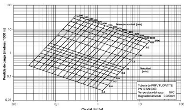
Figura 6-3 Pérdida de carga – diámetros grandes
