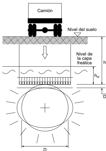
Figura 6-1 Comportamiento del tubo bajo carga de tráfico
