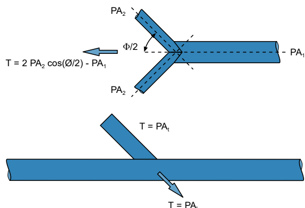
Figura 10-6 Fuerzas de empuje
