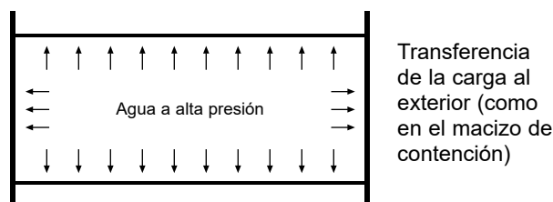
Figura 5-3 Efecto de la presión a largo plazo sobre la vida del tubo
