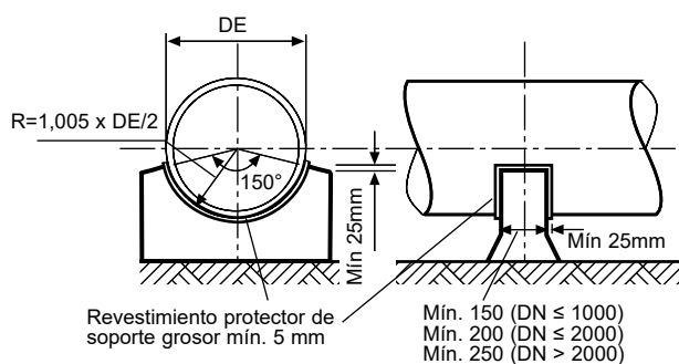
Figura 10-14 Diseño de soportes
