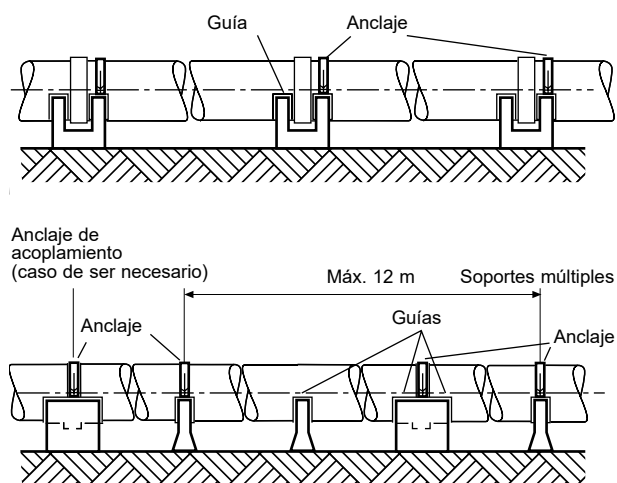
Figura 10-13 Disposición típica de soportes
